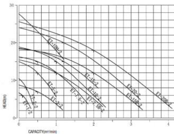
50Hz 4P...1500r/m
