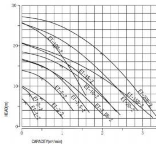
60Hz 4P...1800r/m
